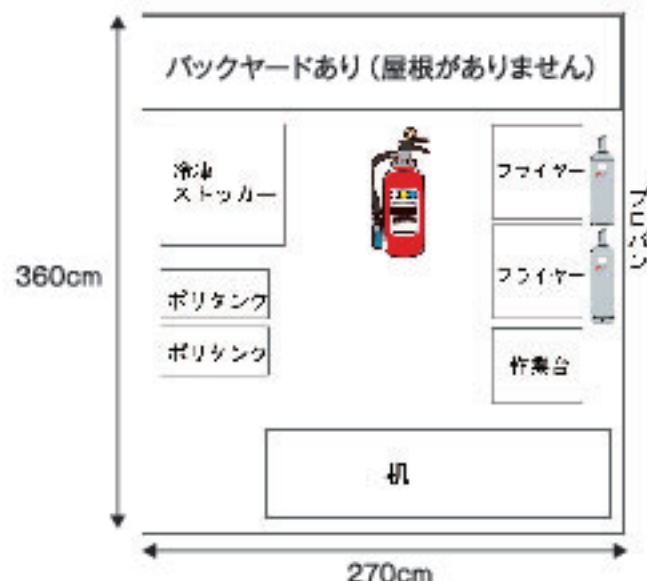
手羽先ブース レイアウト例（平面図）
