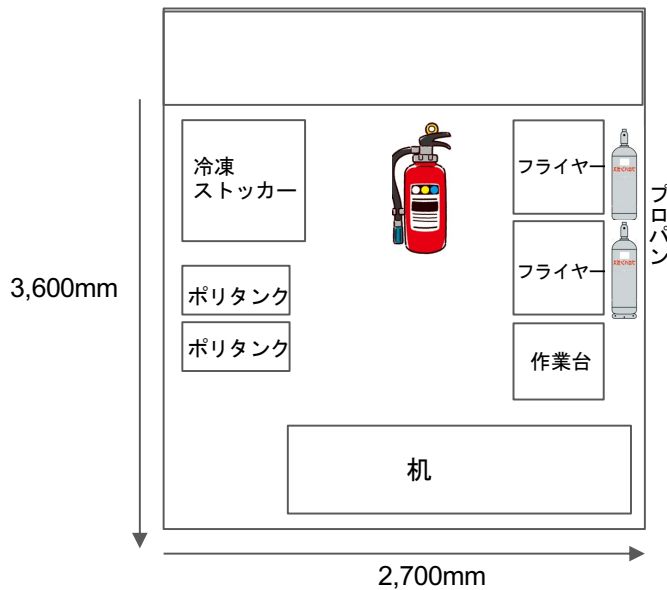
ブースレイアウト例（平面図）
