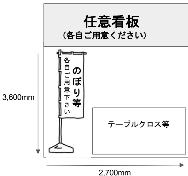
ブースレイアウト例（正面）
